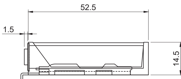
Imán atornillable
