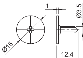
Imán atornillable
