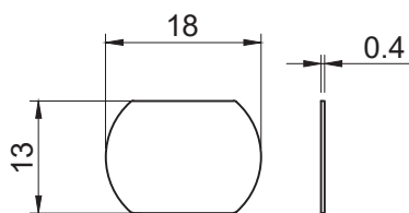
Imán adhesivo
